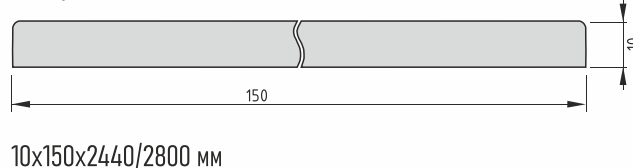
Добор плоский
