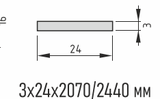
Стыковочная планка
