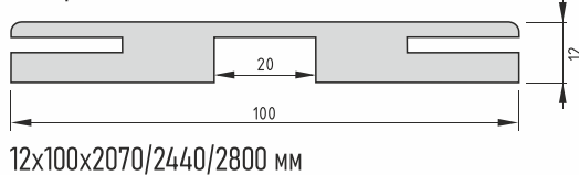
Добор телескопический
