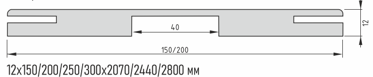
Добор телескопический
